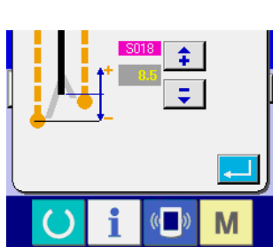
Tela de costura de ajuste de faca de canto (Tela C)
